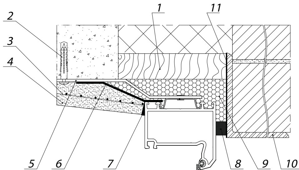
Рисунок 5.5 Узел верхнего примыкания оконного блока к перемычке из стального уголка в проеме многослойной стены с облицовкой кирпичом
