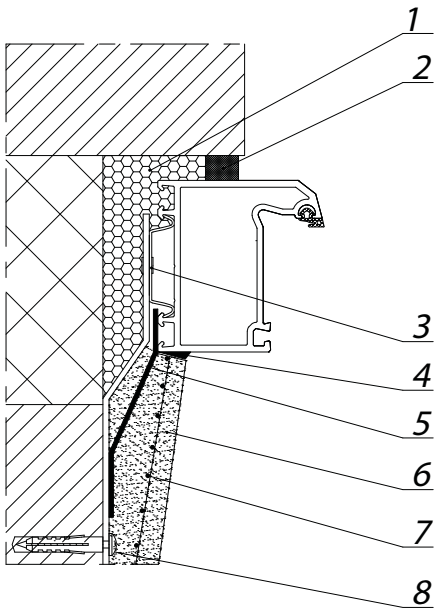
Рисунок 5.3 Узел бокового примыкания оконного блока к проему с четвертью слоистой стены из кирпича с эффективным утеплителем и отделкой внутреннего откоса штукатурным раствором
