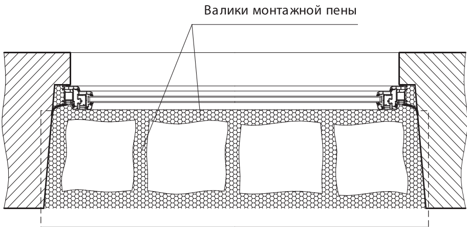
Рисунок 8.1 Схема нанесения монтажной пены в пространство под подоконником
