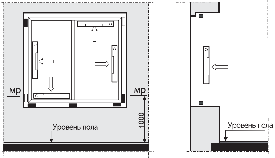
Рисунок 6.1 Схема проверки вертикальности установки оконного блока
