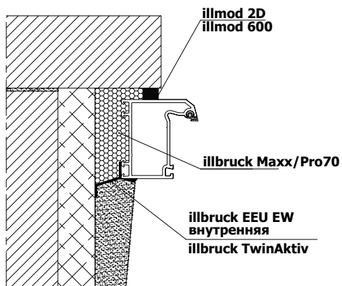
Рисунок 1.1 Боковой и верхний узлы примыкания оконных блоков к стеновым проемам с отделкой внутренних откосов штукатурным раствором.
