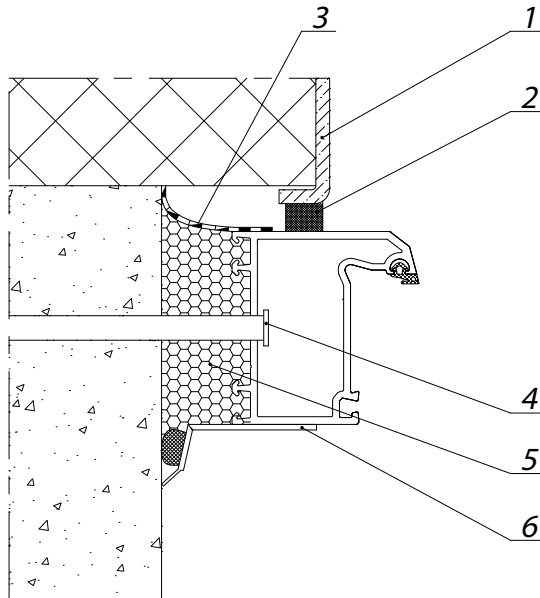
Рисунок 5.8 Узел бокового примыкания оконного блока к проему стены из бетона с наружным утеплением фасада и установкой внутреннего декоративного нащельника пароизоляционной системой
