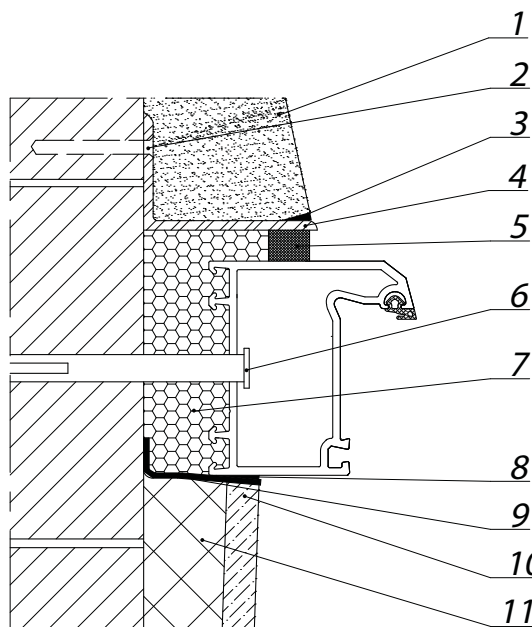
Рисунок 5.2 Узел бокового примыкания оконного блока к проему без четверти в стене из кирпича и отделкой внутреннего откоса облицовочной панелью
