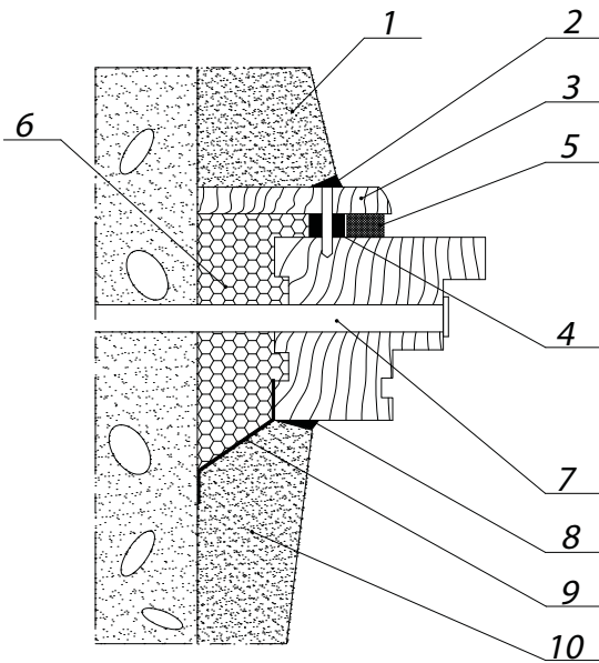
Рисунок 5.7 Узел бокового примыкания оконного блока к проему без четверти в стене из ячеистобетонных блоков с отделкой, наружных и внутренних откосов штукатурным раствором
