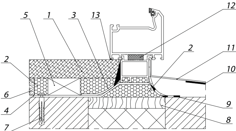
Рисунок 5.4 Узел нижнего примыкания оконного блока, подоконника и слива к проему слоистой стены с эффективным утеплителем
