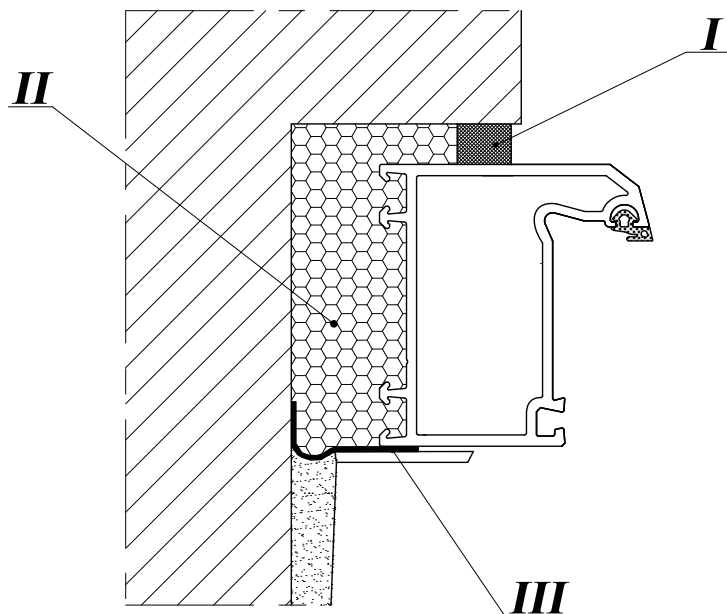
Рисунок 1. Принципиальная схема монтажного шва
