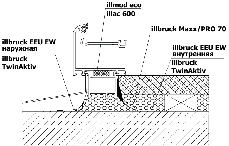
Рисунок 1.3 Нижний узел примыкания оконного блока, подоконника и оконного слива к стеновому проему.
