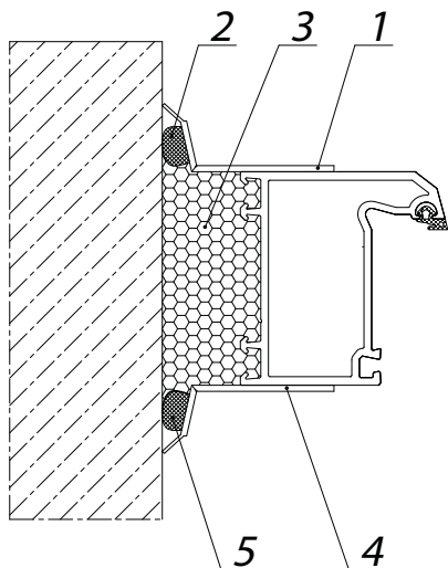
Рисунок 7.1 Узел изоляции и отделки оконного стыка за одну рабочую операцию (планки установлены с наружной или внутренней сторон стыка)
