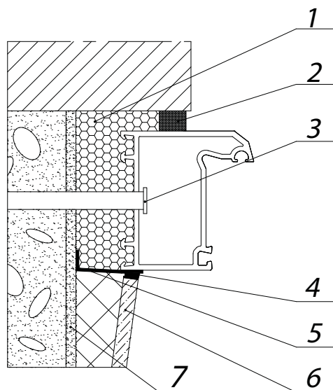
Рисунок 5.6 Узел бокового примыкания оконного блока к проему с четвертью в стене из ячеистобетонных блоков (плотностью 400 – 450 кг/м 3 ) с облицовкой кирпичом и отделкой внутреннего откоса панелью
