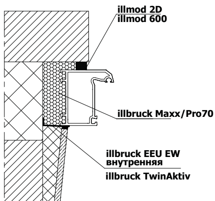
Рисунок 1.2 Боковой и верхний узлы примыкания оконных блоков к стеновым проемам с отделкой внутренних откосов панелями.
